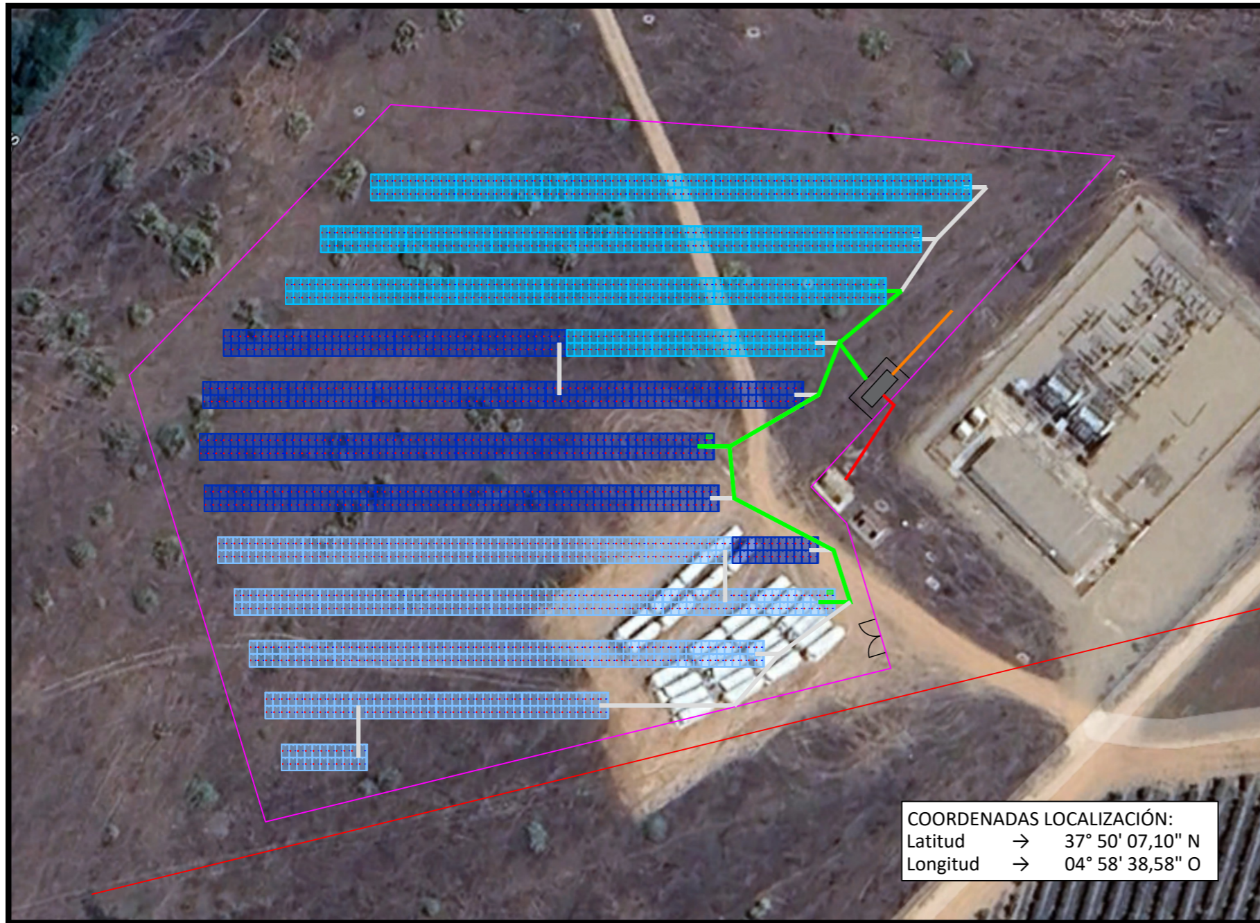
B IMPLANTACIÓN GENERAL E: 1:900
